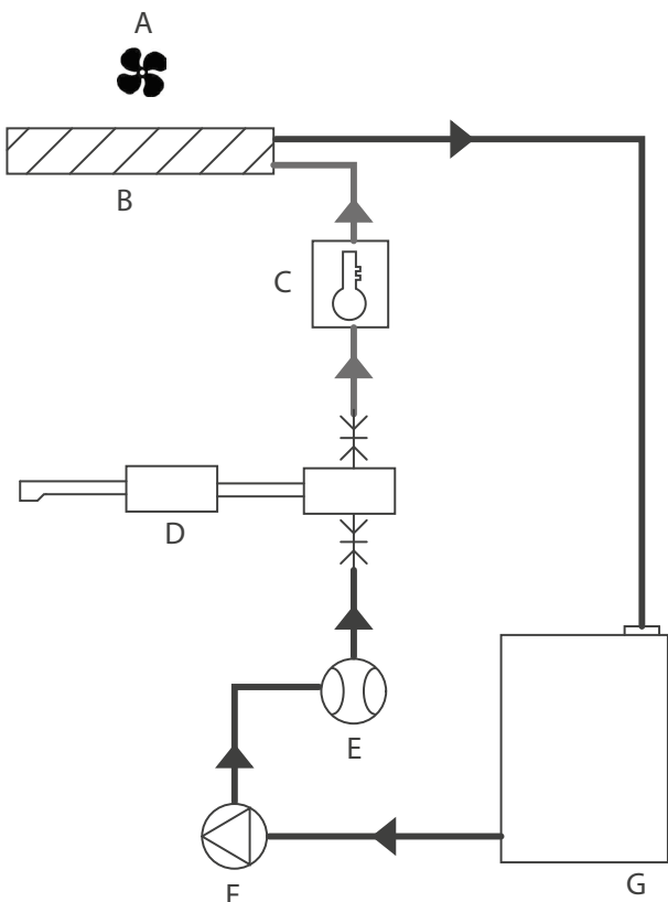
DIAGRAMME DU CIRCUIT DE REFRIGERISSEMENT / COOLING CIRCUIT DIAGRAM / DIAGRAMA DEL CIRCUITO DE REFRIGERACION / ДИАГРАММА ЦЕ ПИ ОХЛАЖДЕНИЯ / SCHEMA KOELCIRCUIT / DIAGRAMMA DEL CIRCUITO DI RAFFREDDAMENTO
